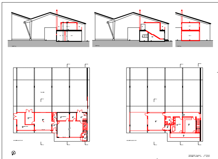
Grundrisse Forstgebäude
